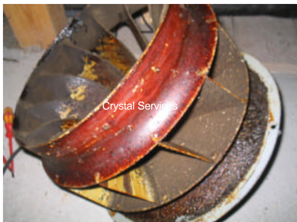
Ventilatorrad vorher
